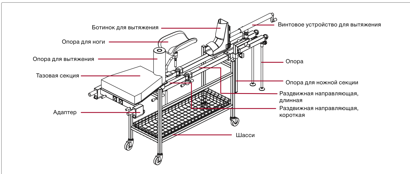
Ортопедическая система для вытяжения 115-005691(005778PU)-00
