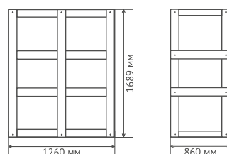
Габаритные размеры в деревянной обрешётке, мм
