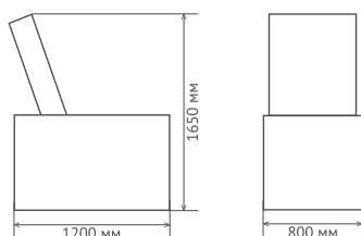
Габаритные размеры в гофрокартонной упаковке, мм
